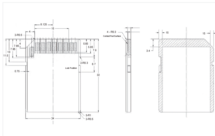
Méretek mm-ben
