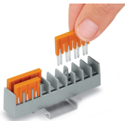
Áthidaló gyűjtő Áthidaló behelyezése.
