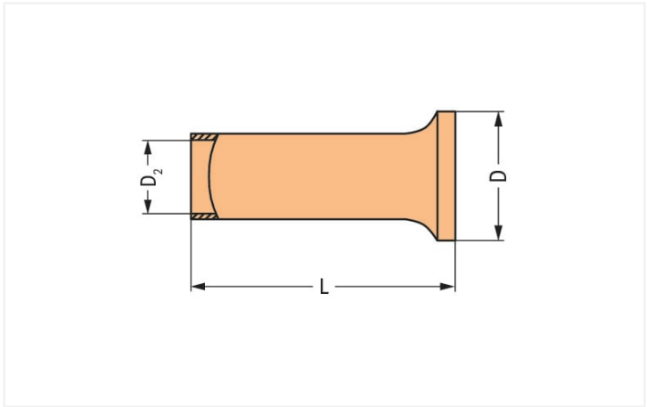
Méretetek mm-ben
